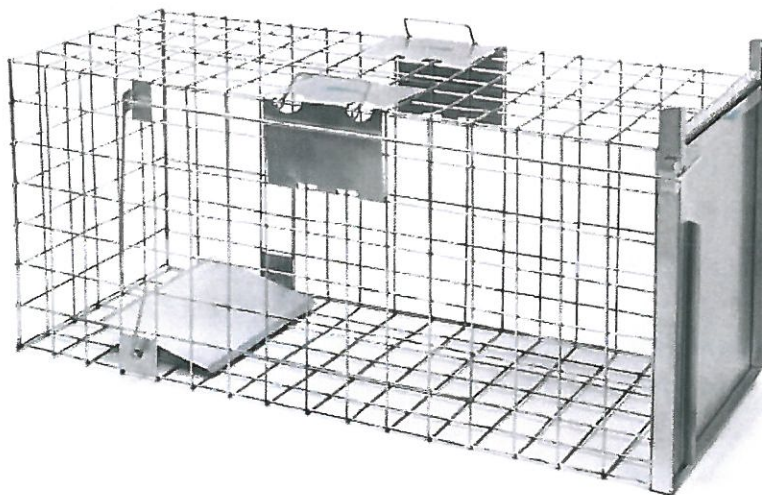
Fot. 4 Przykładowy wygląd pułapki jednostronnej o wymiarach 118-122 cm dł. 38-41 cm szer. i 48-51 cm wys.
