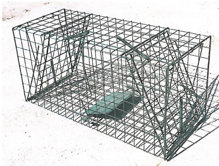
Fot. 3 Przykładowy wygląd pułapki dwustronnej o wymiarach 118-122 cm dł. 49-51 cm szer. i 55-58 cm wys.
