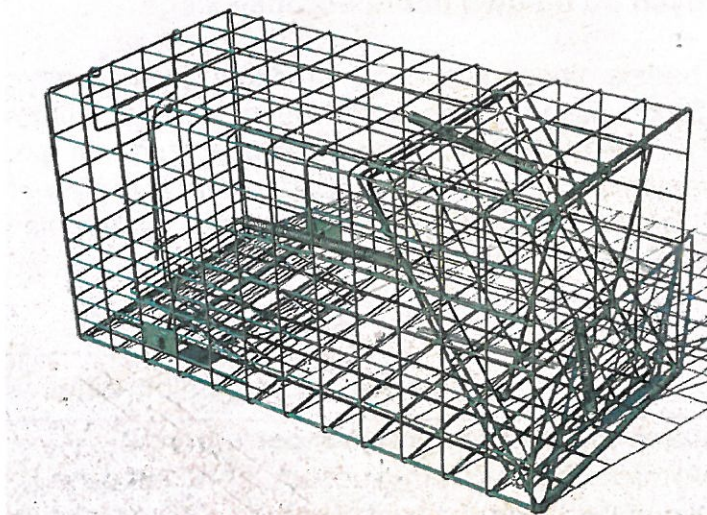
Fot. 2 Przykładowy wygląd pułapki jednostronnej o wymiarach 83-86 cm dł. 40-43 cm szer. i 40-43 cm wys.
